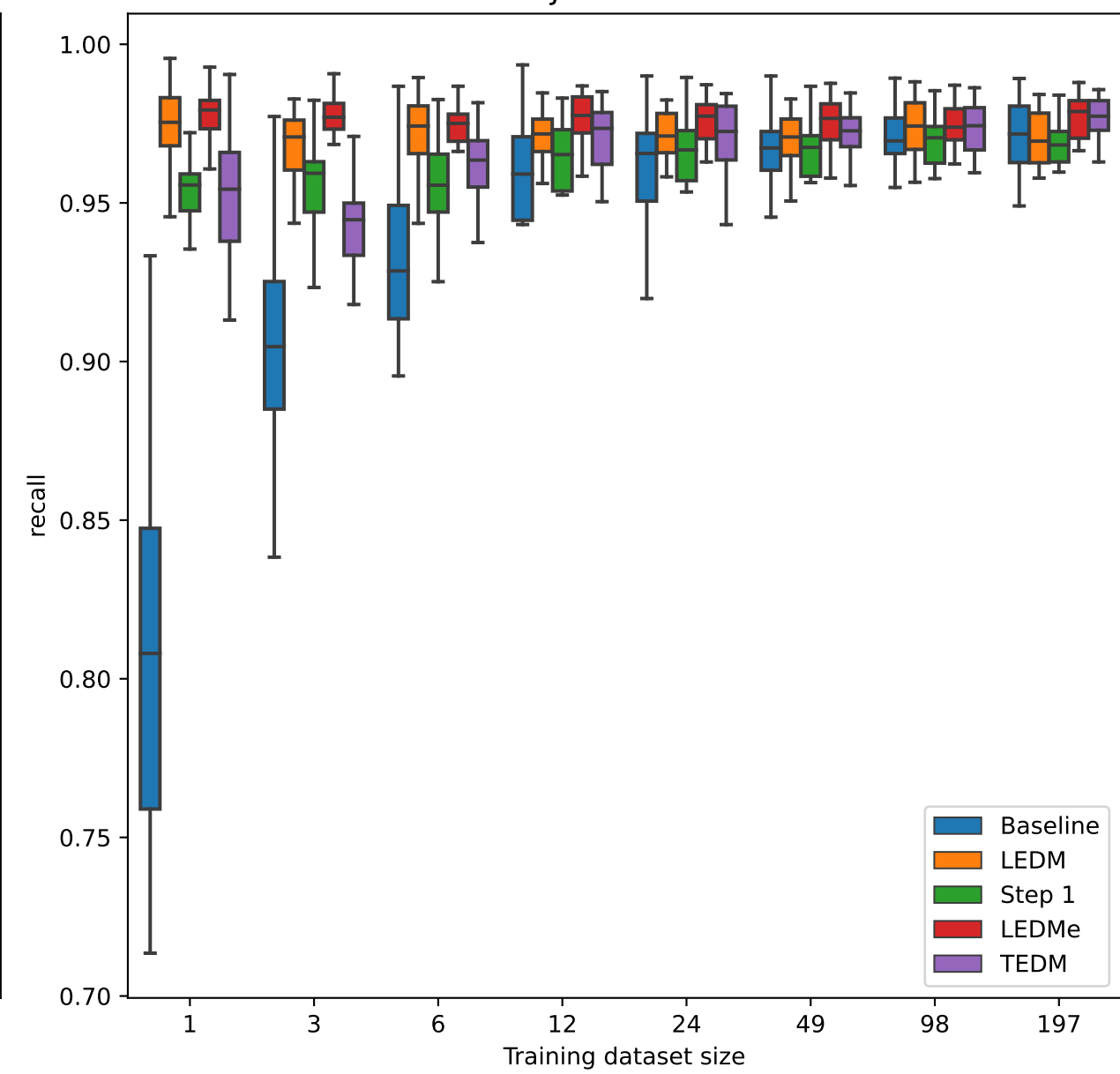
NIH recall
