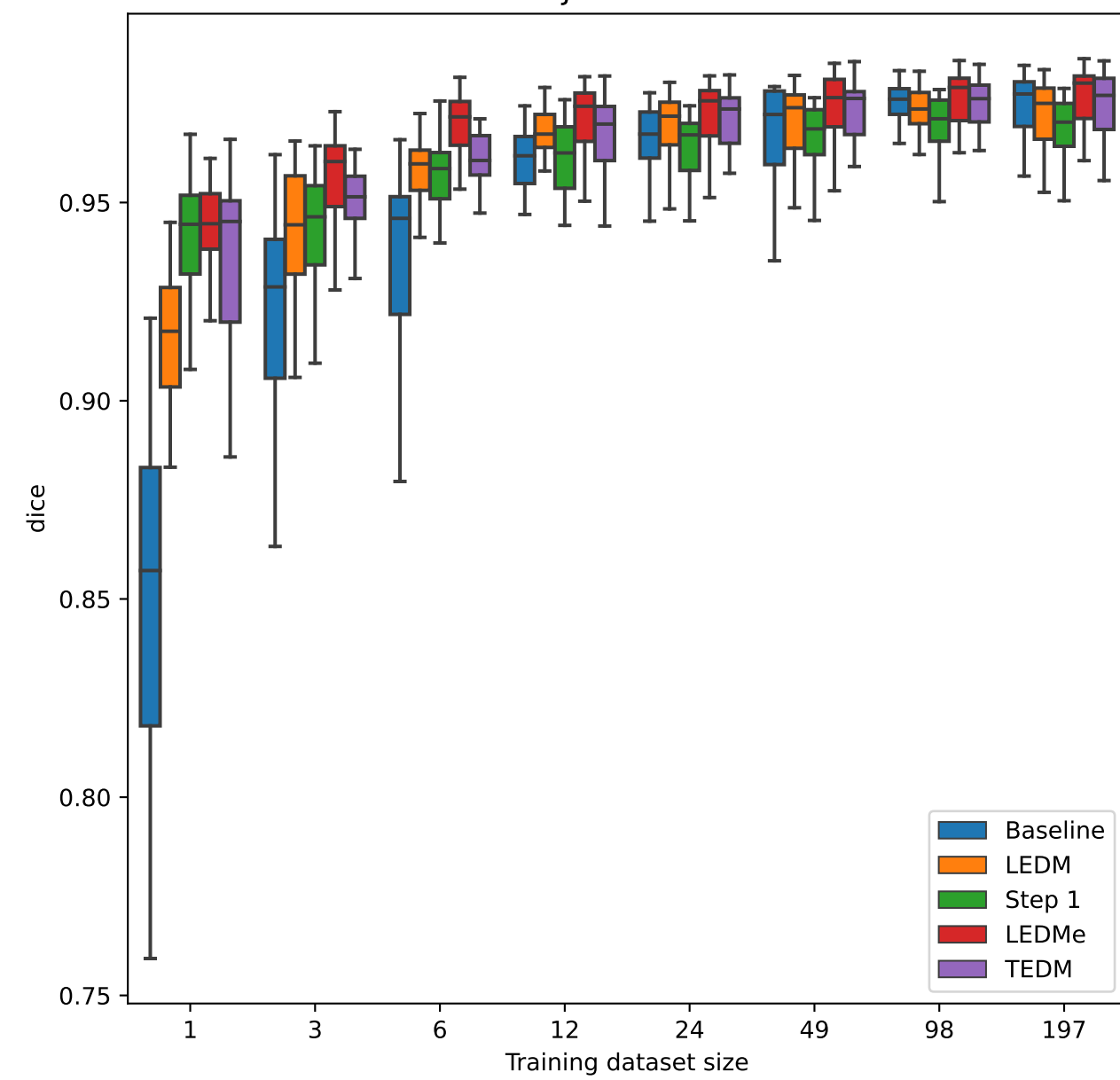
NIH dice
