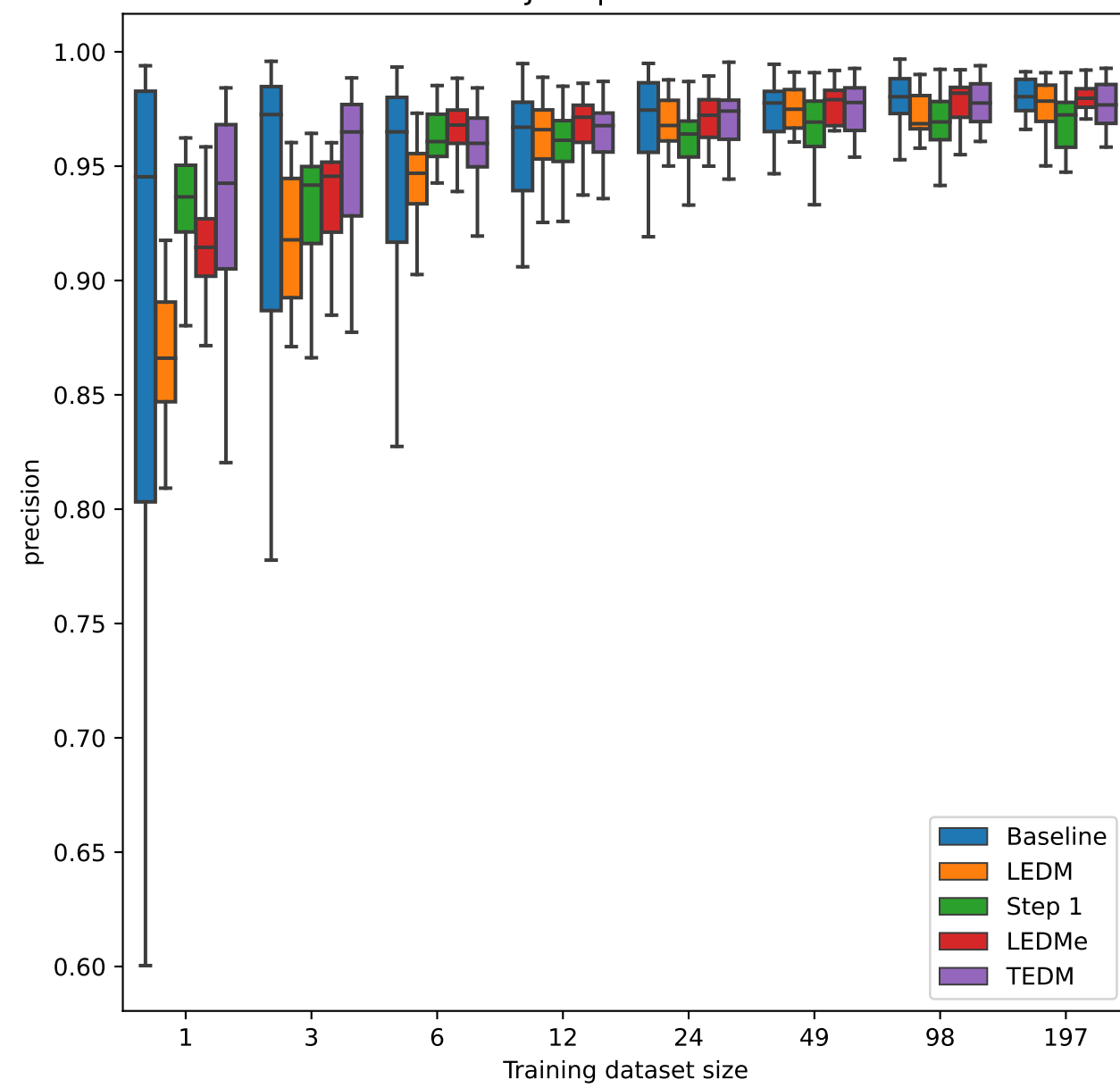
NIH precision
